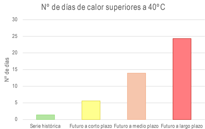
Figura 39. Diagrama de variación del número de días en los que se superan los 40 °C al año en El Cuervo de Sevilla para la serie histórica de 1961 a 1990 y para los horizontes temporales de futuro a corto, medio y largo plazo.
