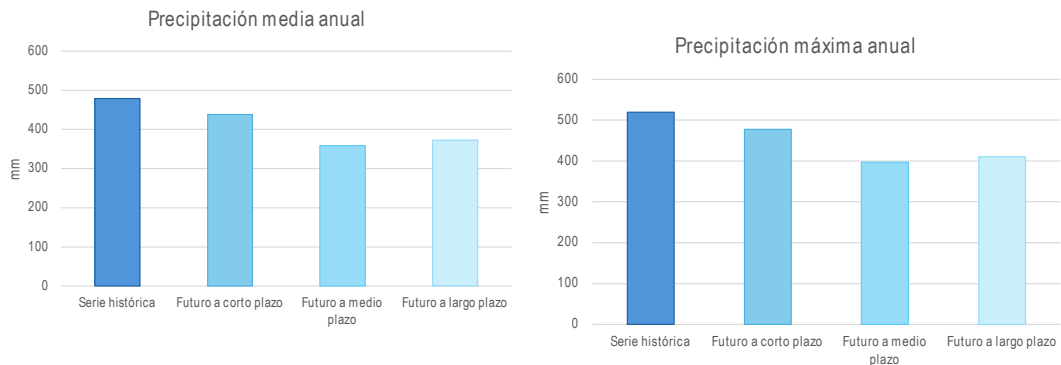
Figura 40. Diagramas de variación de los valores de precipitación media (izquierda) y máxima (derecha) anuales en El Cuervo de Sevilla para la serie histórica de 1961 a 1990 y para los horizontes temporales de futuro a corto, medio y largo plazo.
