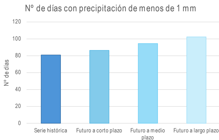
Figura 42. Diagrama de variación del número de días al año en los que se registran en El Cuervo de Sevilla valores de precipitación inferiores a 1 mm para la serie histórica de 1961 a 1990 y para los horizontes temporales de futuro a corto, medio y largo plazo.
